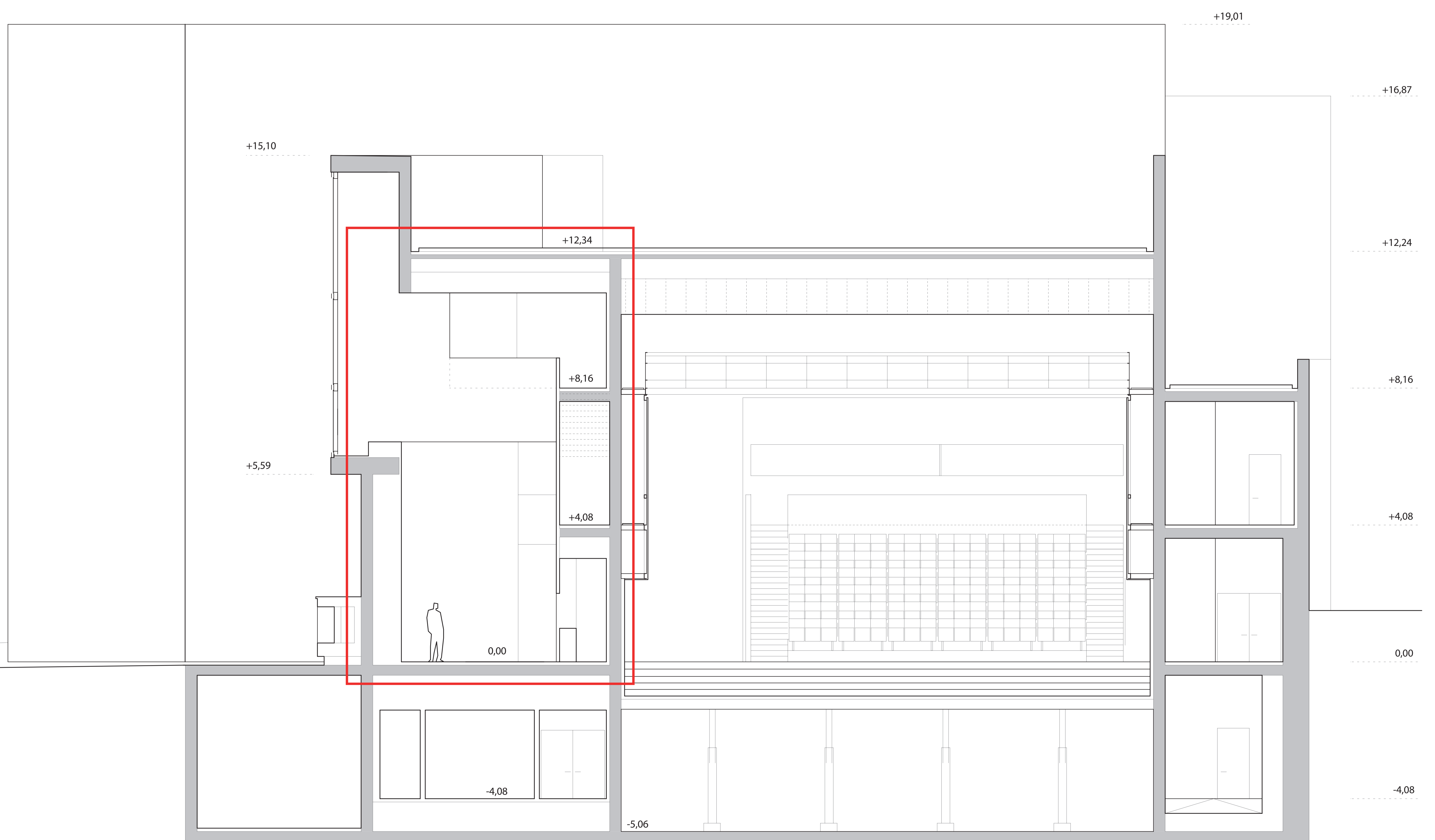
SECCIÓN TRANSVERSAL POR VESTÍBULO
