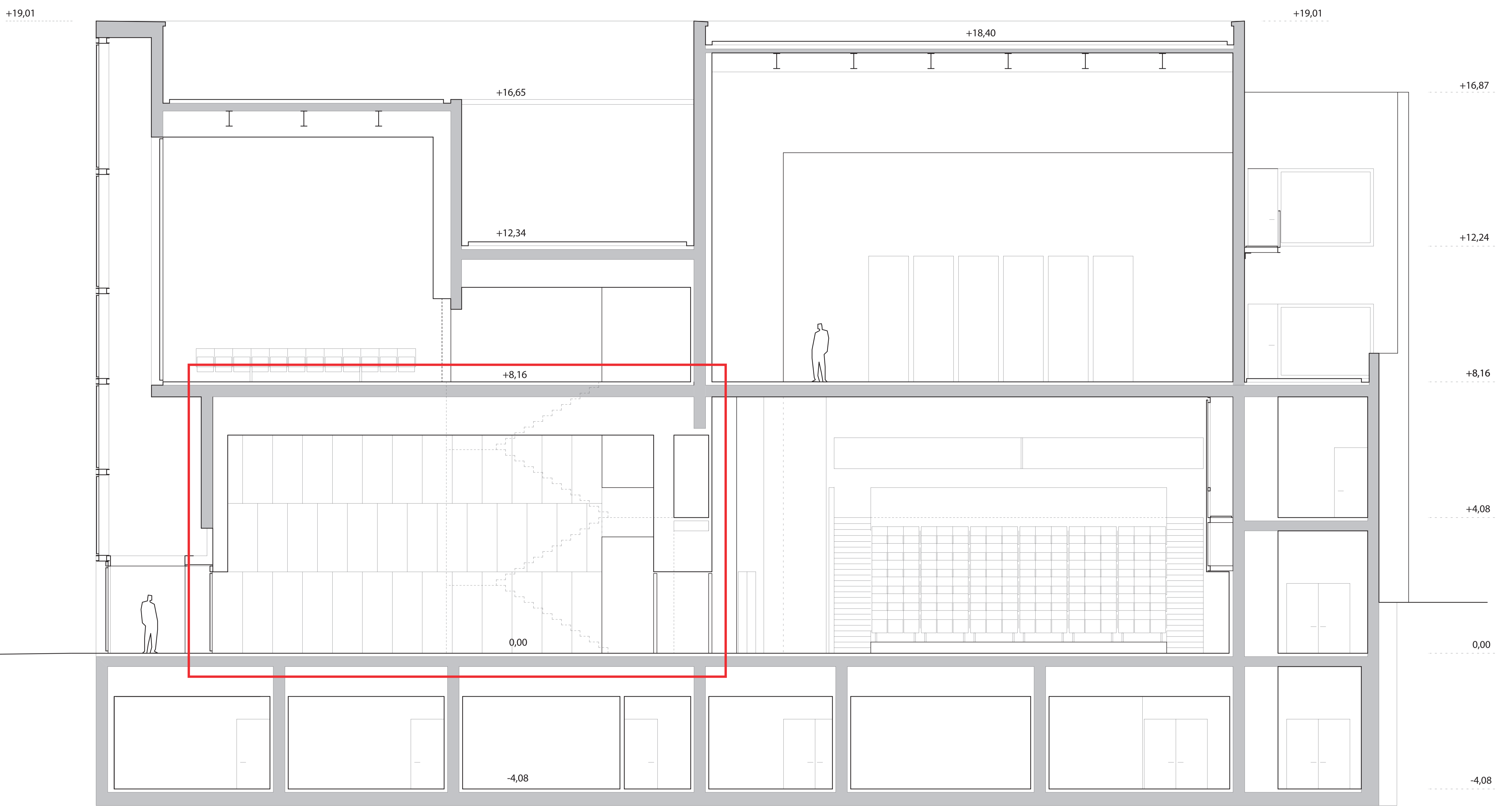
SECCIÓN TRANSVERSAL POR SALAS
